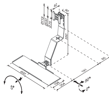
HM-005 连接头与键盘托盘
