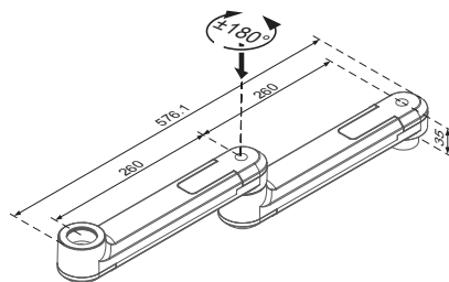
HM-052 手臂
