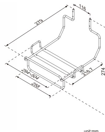
HAA-11 键盘托架
