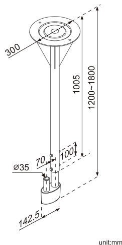
HA-237P 天花板安装
